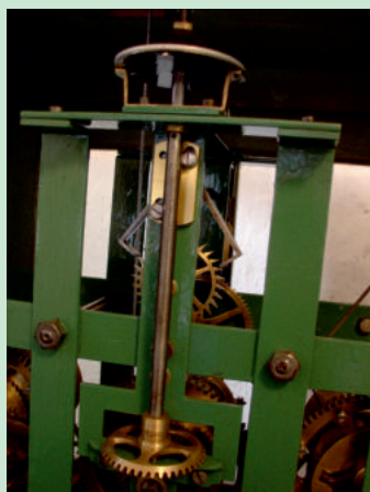
Svislý převod na náhon ruček s kužlovým soukolím, nahoře pomocný minutový číselník, krokové kolo s kotvou a posuvné ložisko, Nahořany, kaple Sv. Rodiny, věž;
